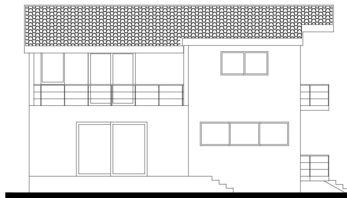
PROSPETTO ANTERIORE
