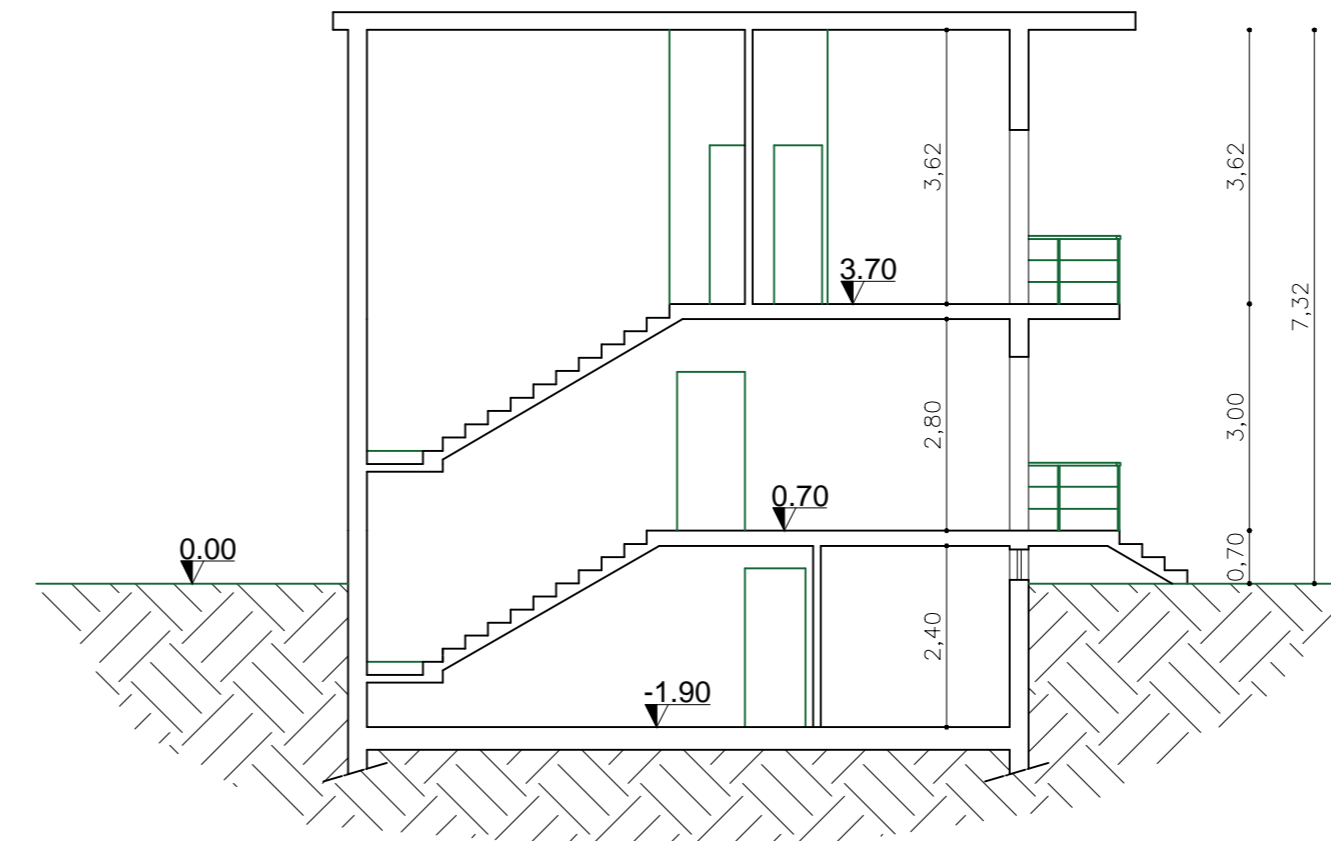
SEZIONE A-A
