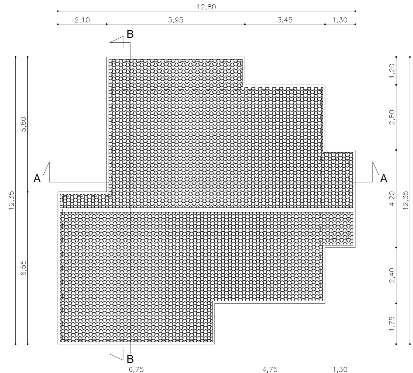
PIANTA COPERURE
